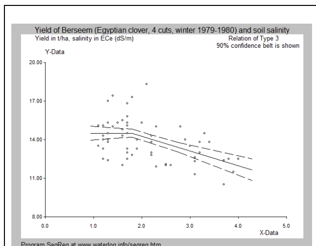
Fig. 2.1 Berseem. BP=1.8 dS/m
