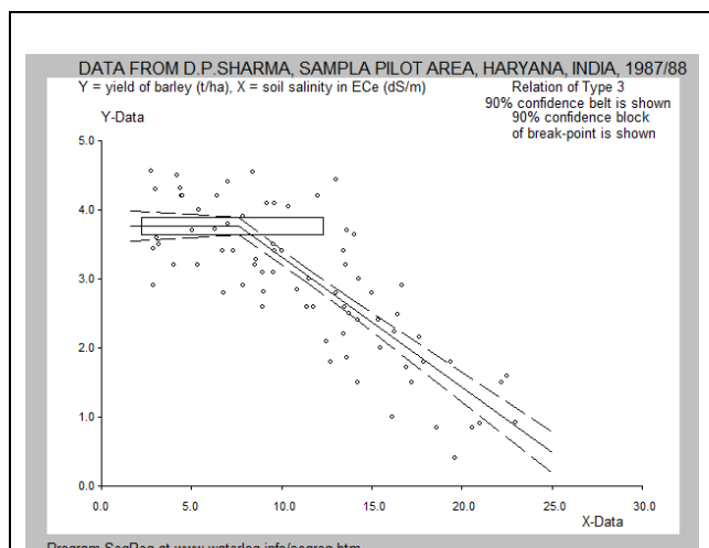
Fig. 4.1 Barley. BP=7.6 dS/m
