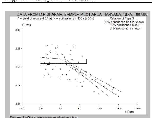
Fig. 4.2 Mustard (rapeseed). BP=5 dS/m
